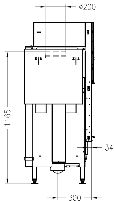
Seitenansicht M~1:20
